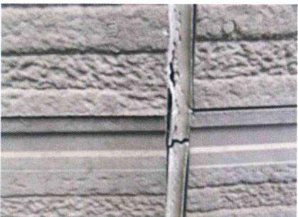
シーリング(コーキング)が経年によって劣化し、痩せて裂け目が入ってきています。
