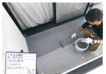
ウレタン防水(オートンエナガード)のトップコートを塗布していきます。
